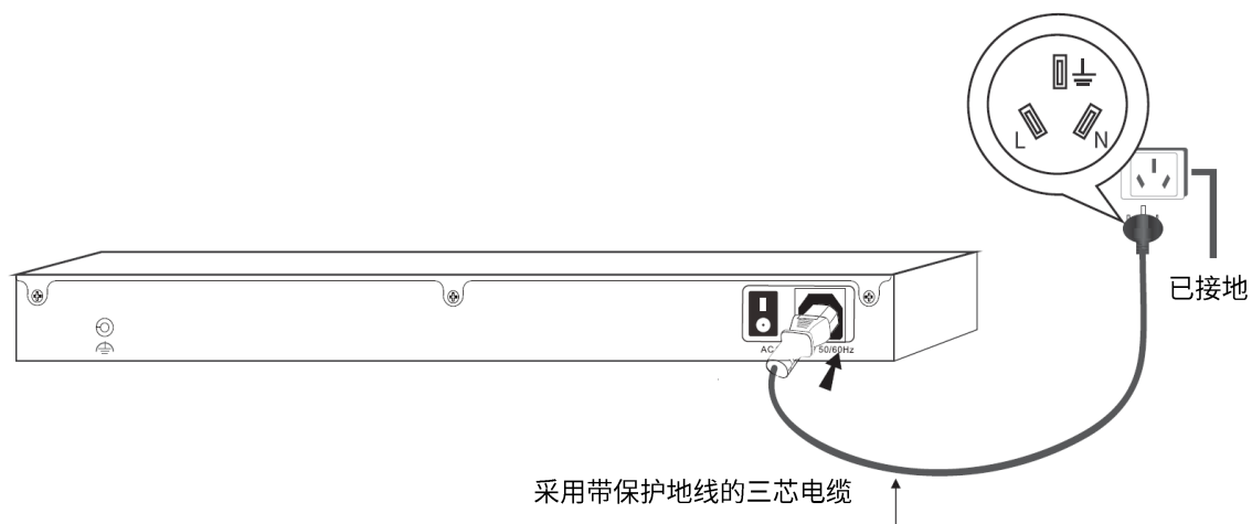
图 2-3 通过电源线接地
