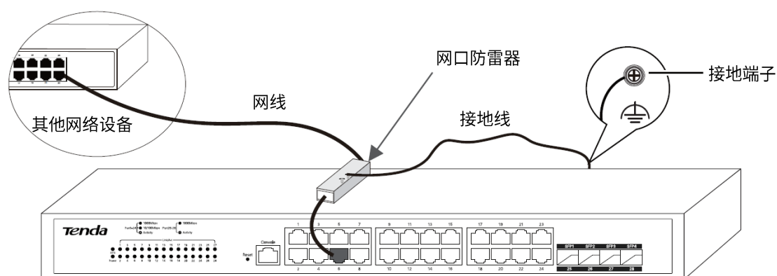
图 3-1 连接网口防雷器
