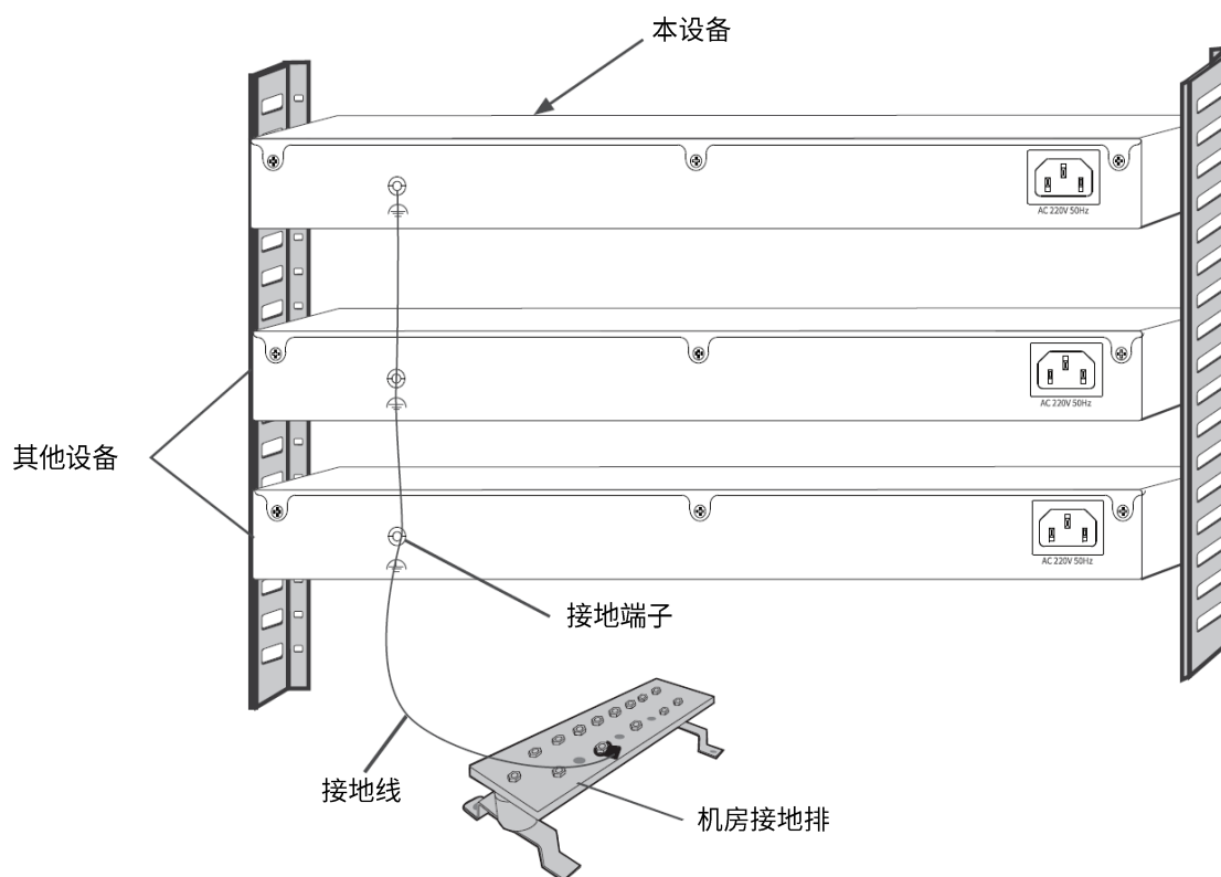
图 2-4 等电位连接简图
