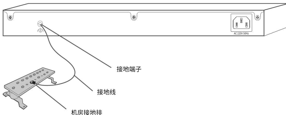
图 2-1 机房有接地排时接地安装简图
